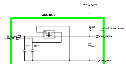
19.2MHz OSC
